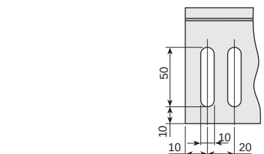
THIN SLOT
